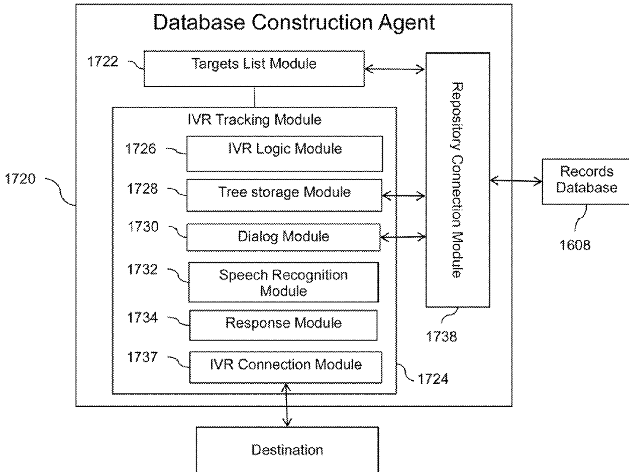
FIG. 17C
