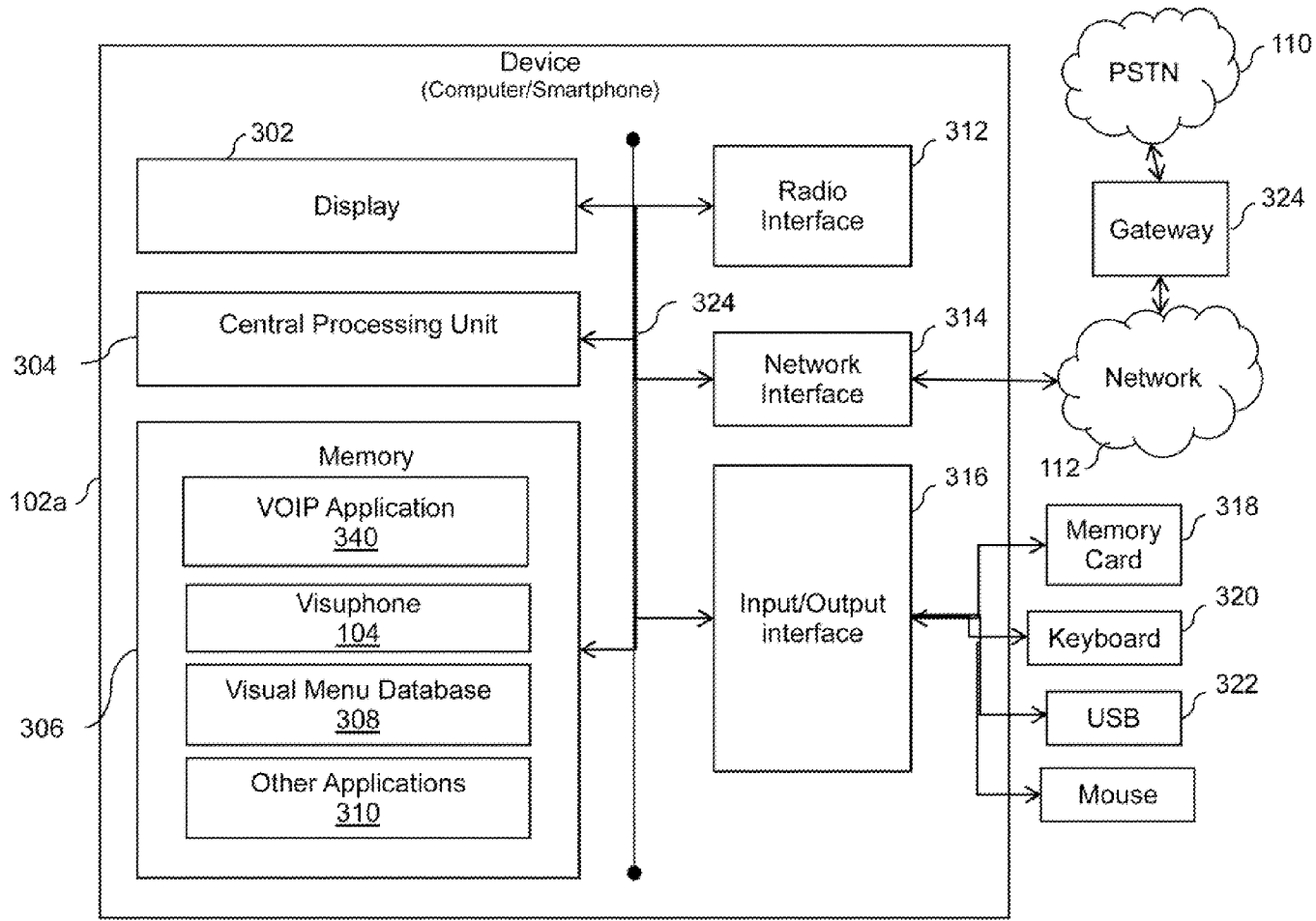
FIG. 3B
