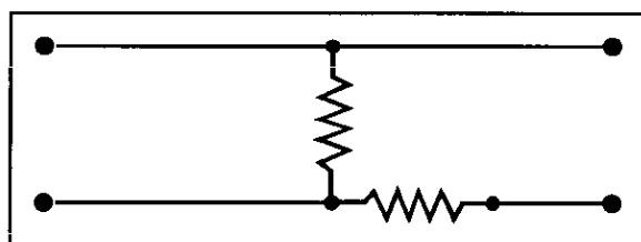
L-pad
